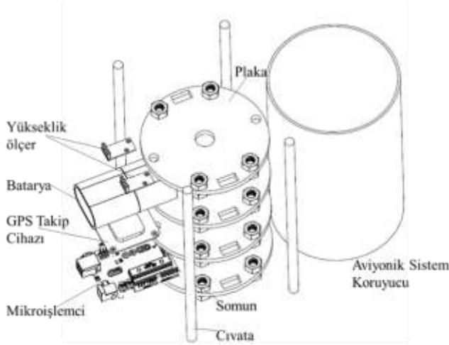
Görsel 7. Aviyonik Sistem Montaj Resmi
