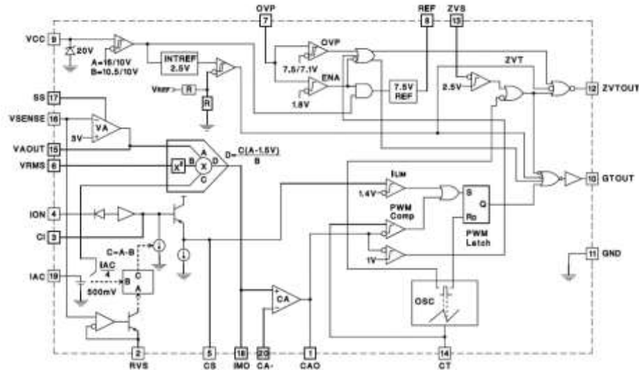
Görsel 10 UC3855 Devre Şeması
