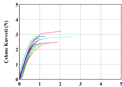
200-210-220-230-240-245 °C 'nin her blümünde 20 dk beklemeli viskoz rayon
