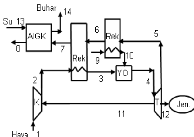
Görsel 2. Gaz türbinli yakıt hava ısıtımli kojenerasyon şeması
