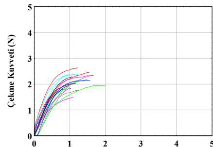
200-210-220-230-240-245 °C 'nin her blümünde 30 dk beklemeli viskoz rayon
