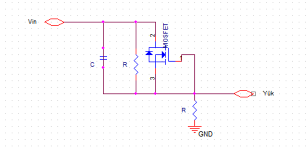
Görsel 9 Inrush Protection Devresi
