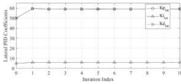
Görsel 6. Her yinelemede yanal PID
