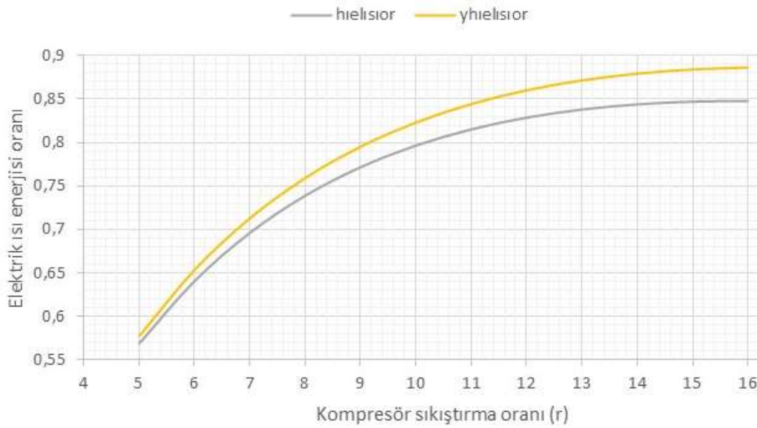
Görsel 8. Elektrik ısı enerjisi oranının kompresör sıkıştırma oranı ile değişimi
