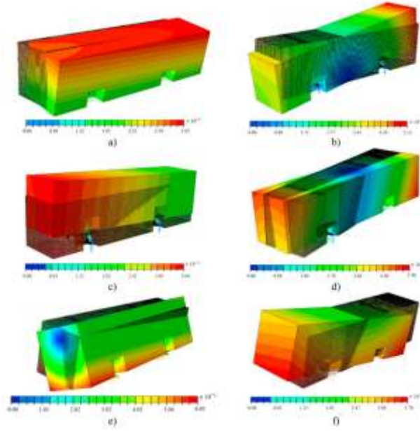
Görsel 9. 12 m uzunluğundaki bir otobüs yapısının modal analiz sonuçları [15]
