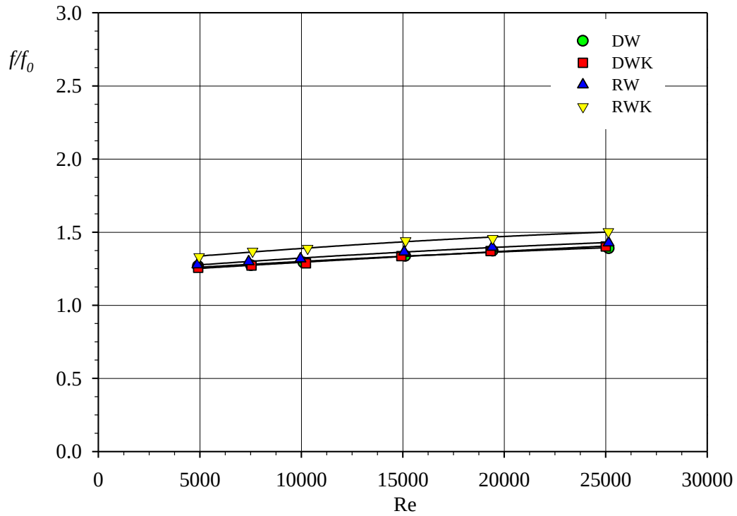
Görsel 7. Boş kanala göre sürtünme faktöründeki artış oranlarının Re ile değişimi
