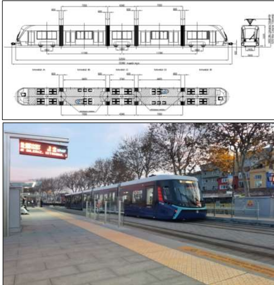
Görsel 4. T5 tramvay hattında kullanılan araç
