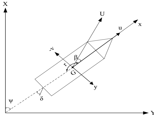
Görsel 1. Gemi ekseni ile yer ekseninin gösterimi.
