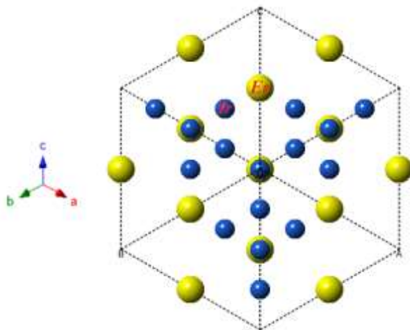
Görsel 1. ErIr 2 bileşiğinin C15-tipi kübik kristal yapısında 3-uzanımlı görüntüsü
