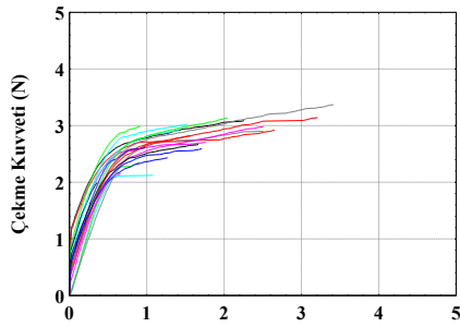
200-210-220-230-240-245 °C 'nin her blümünde 15 dk beklemeli viskoz rayon
