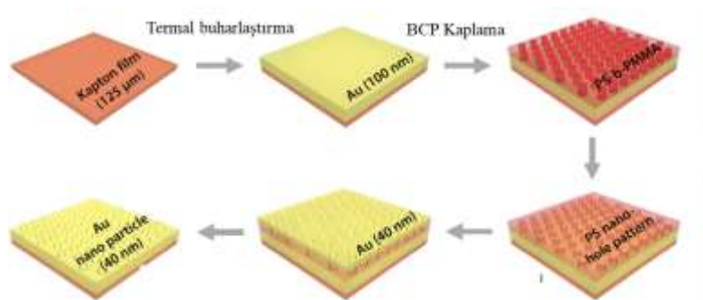
Görsel 3. Blok kopolimer yardımıyla geliştirilen altın (Au) yapıli nanojeneratör üretim sürecinin şematik gösterimi [8]
