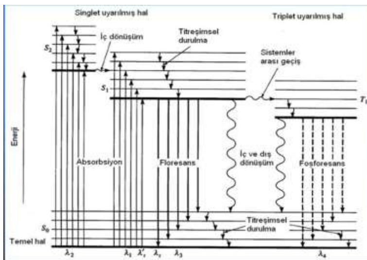
Görsel 1. Bir Fotolüminesans Sistem; Absorbsiyon, Fluoresans ve Fosforesans İçin Kısmi Jablonski (Enerji) Diyagramı [6]
