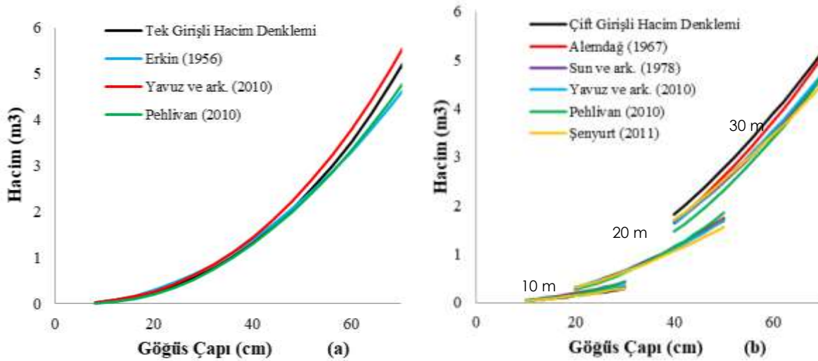
Görsel 2. Sarıçam tek girişli ağaç hacim eğrilerinin karşılaştırması
