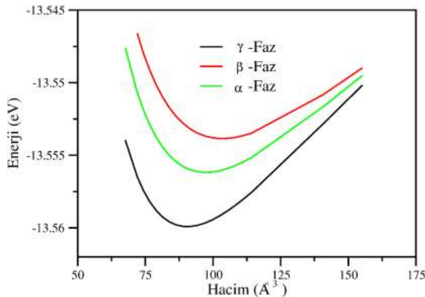
Görsel 1. NdPdBi Yarı-Heusler Bileşiğinin \alpha , \beta ve \gamma Fazları İçin Toplam Enerji-Hacim Değişimleri
