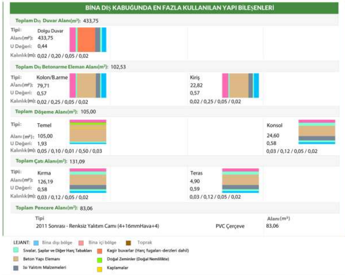
Görsel 8. Örnek Yeni Binaya Ait Bina Dış Kabuğunda En Fazla Kullanılan Yapı Bileşenleri ( duvar,dış betonarme, kiriş döşeme, çatı, pencere) ve lejant BEP- TR Bilgileri
