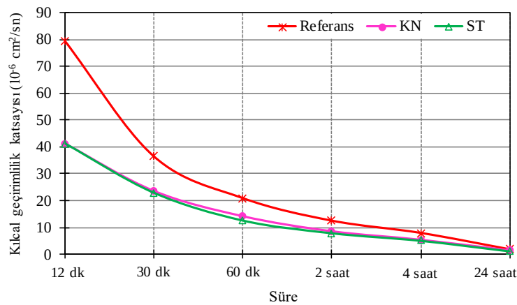
Şekil 2. 12 saat -5 °C'de bekletilen numunelerin kılcal geçirimlilik katsayısının zamana bağlı değişimi
