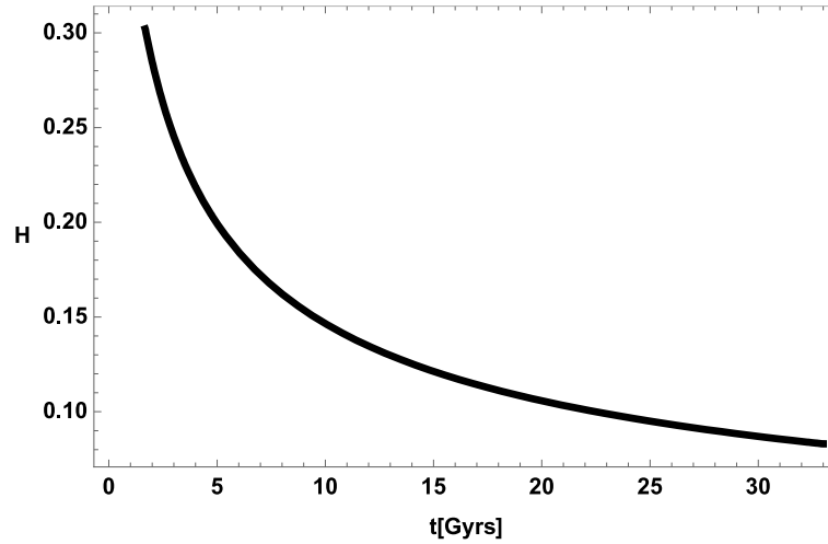
Görsel 1. Hubble parametresinin zamana göre değişimi
