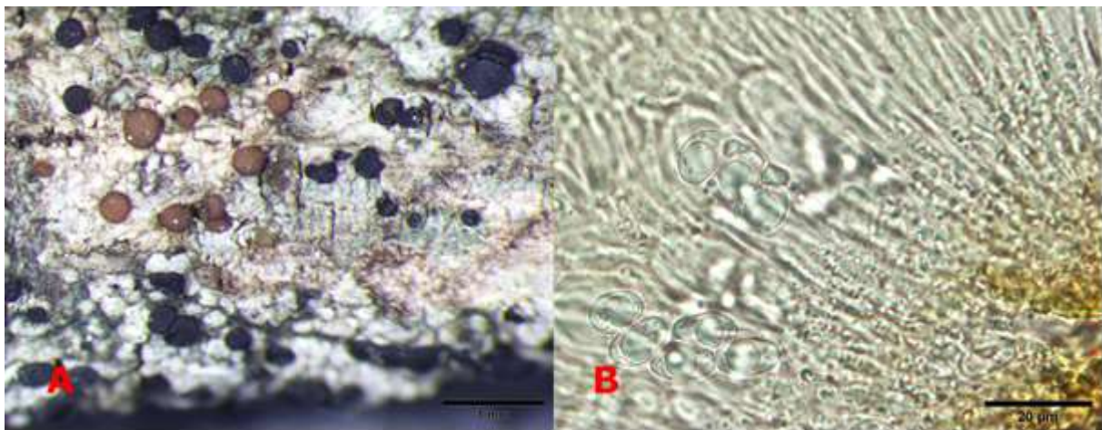
Görsel 1. Protoblastenia terricola taksonunun A. Tallusu, B. Askosporları
