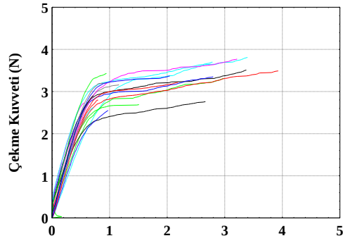
200-210-220-230-240-245 °C 'nin her blümünde 10 dk beklemeli viskoz rayon
