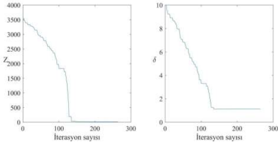
Görsel 6. Hedef 2 için amaç fonksiyonunun ve en iyi dümen açısının iterasyonlar boyunca değişimi.
